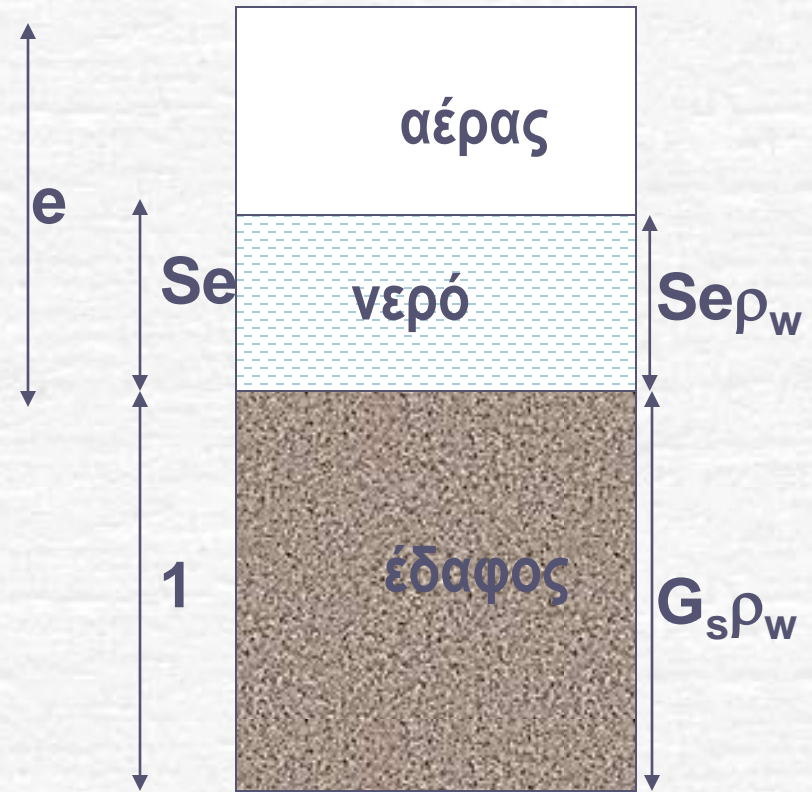
Διάγραμμα Φάσεων
